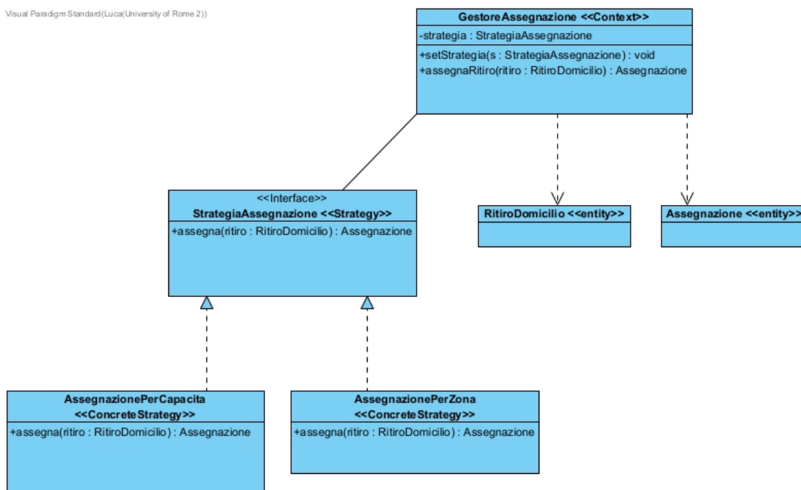
Figura 52: Struttura UML del Design Pattern Strategy per l'allocazione delle risorse
