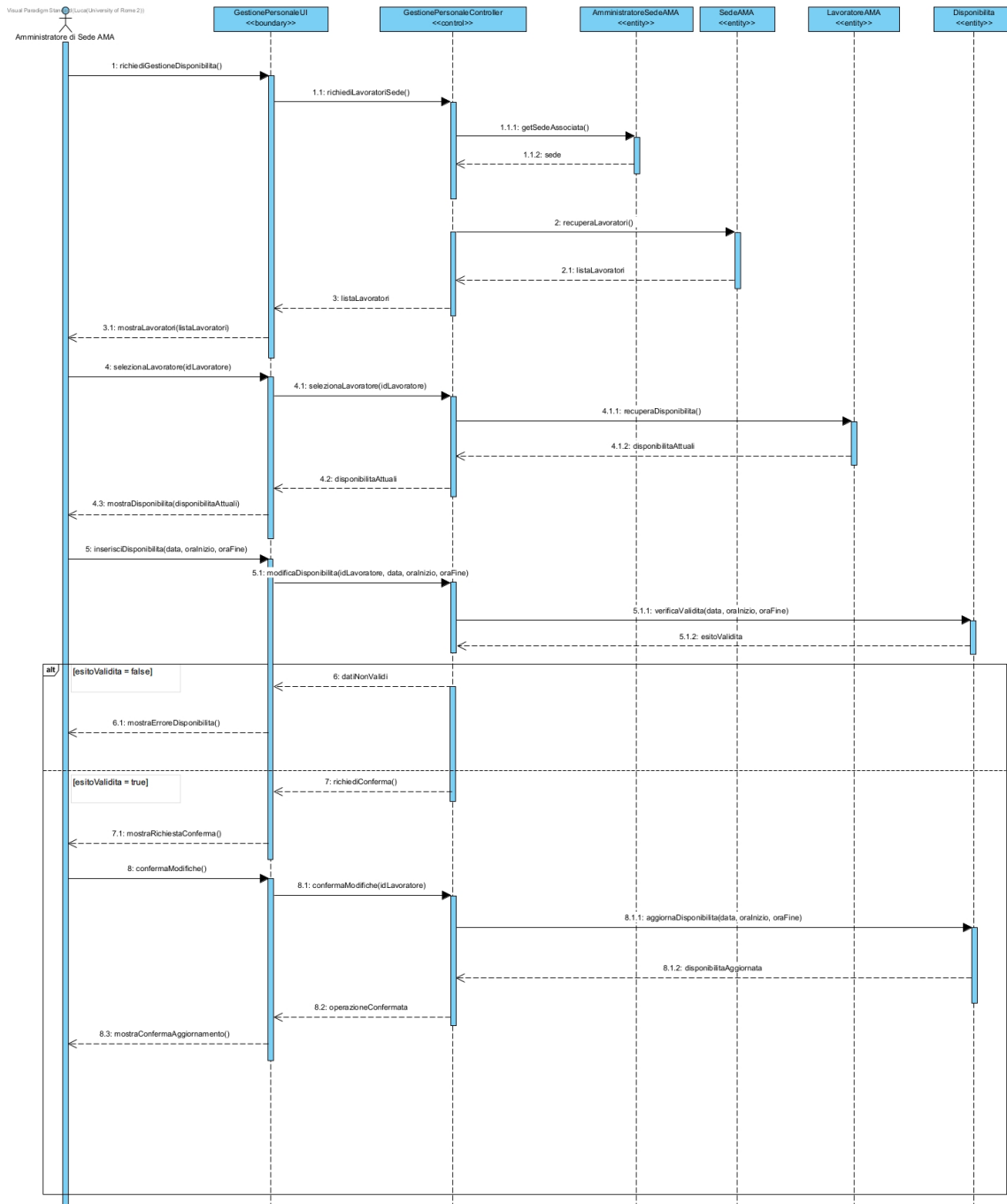
Figura 42: Sequence Diagram — Gestire disponibilità dei lavoratori
