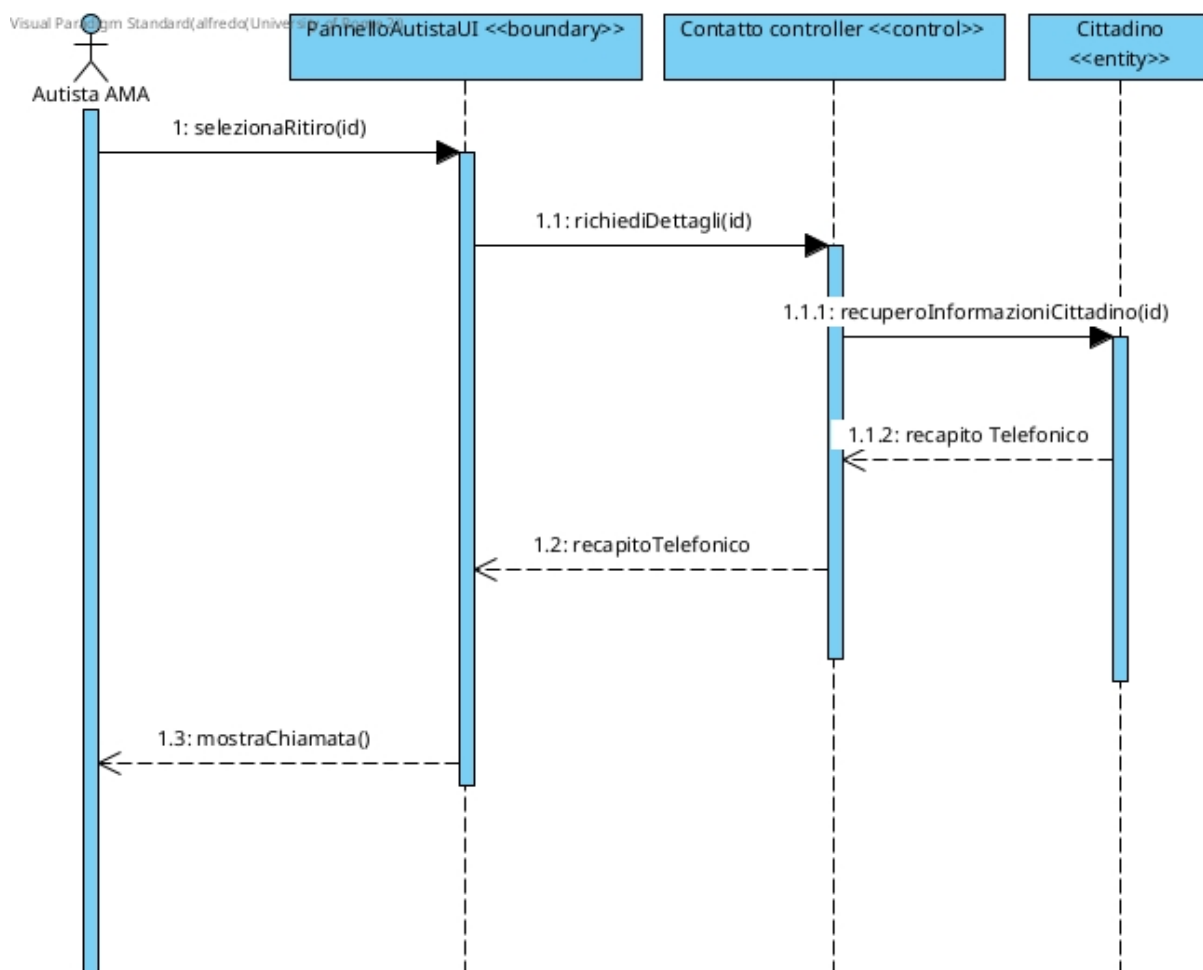
Figura 37: Sequence Diagram — Chiamare cittadino
