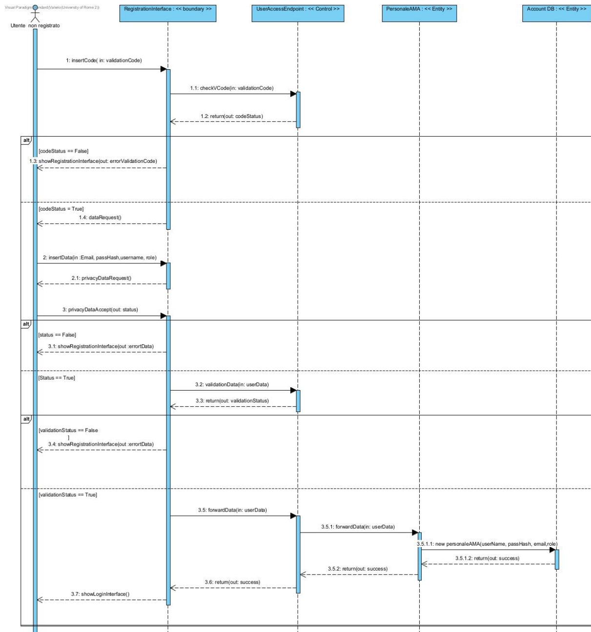
Figura 27: Sequence Diagram — Registrarsi tramite codice di invito
