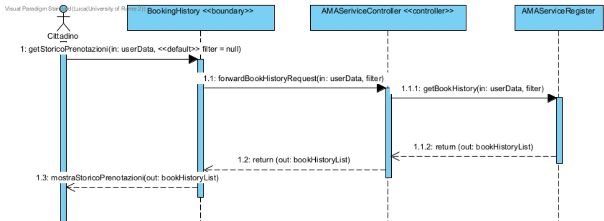
Figura 33: Sequence Diagram — Visualizzare storico prenotazioni
