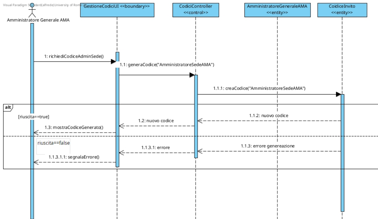
Figura 47: Sequence Diagram — Generare codice amministratore di sede
