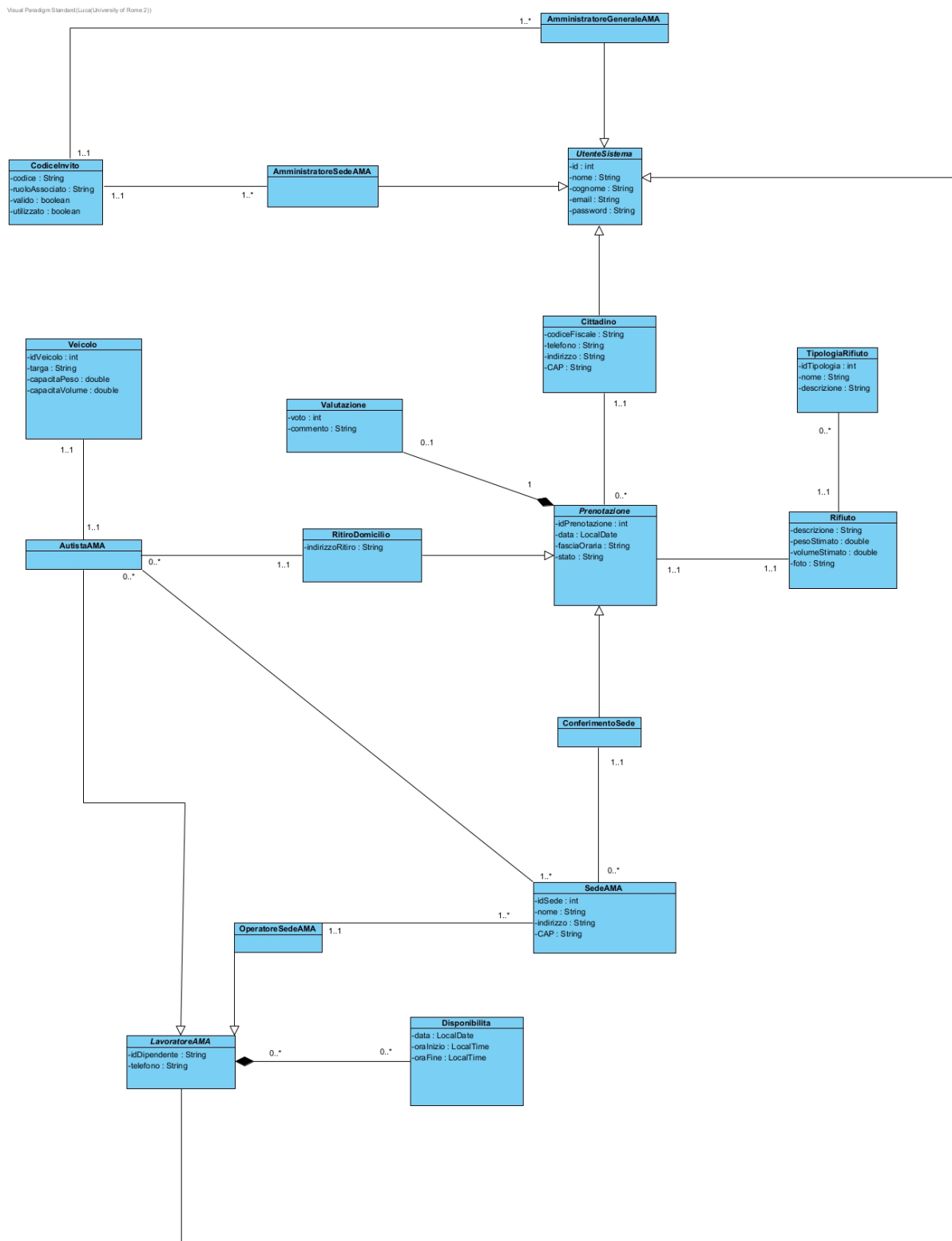
Figura 49: Class Diagram — Versione Unrefined (Modello di Dominio)
