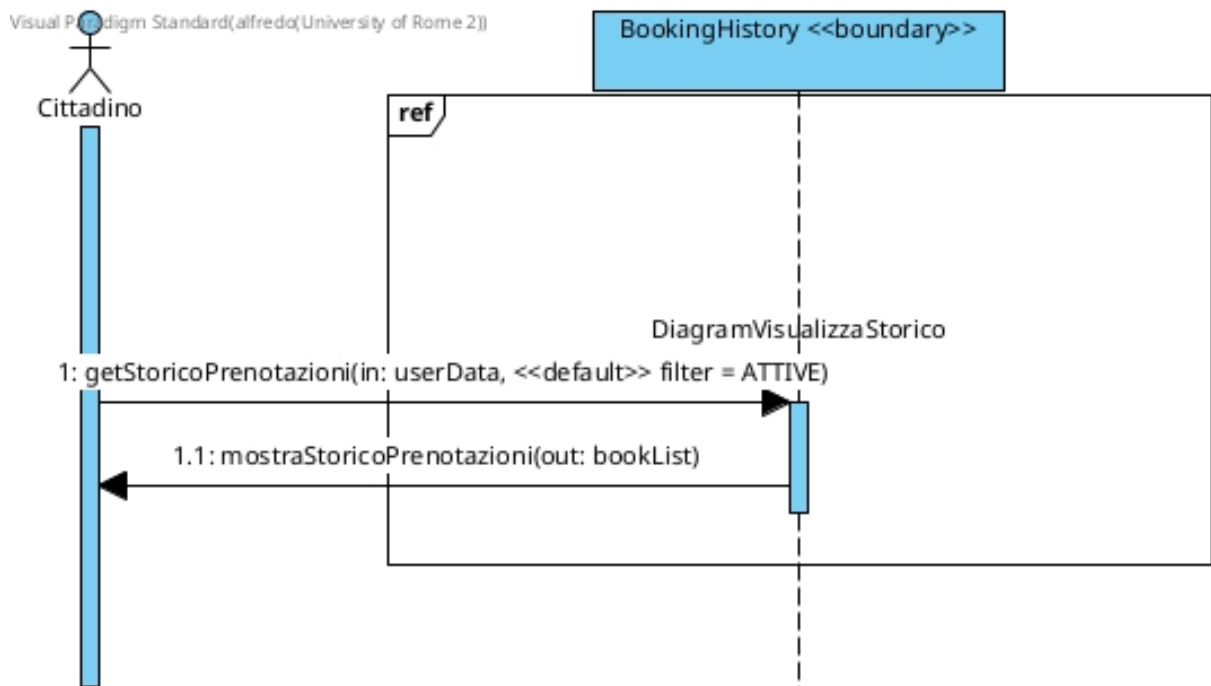
Figura 31: Sequence Diagram — Visualizzare prenotazioni attive
